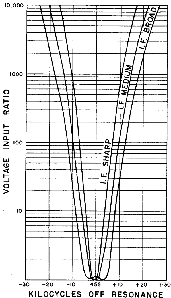
FIG. 1—I. F. SELECTIVITY
